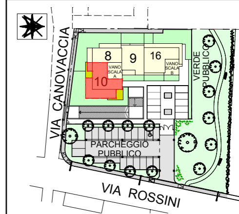
Planimetria generale
