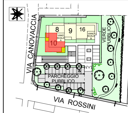
Planimetria generale
